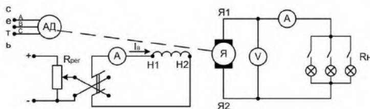
Рис. 1.1. Схема исследования генератора независимого возбуждения
